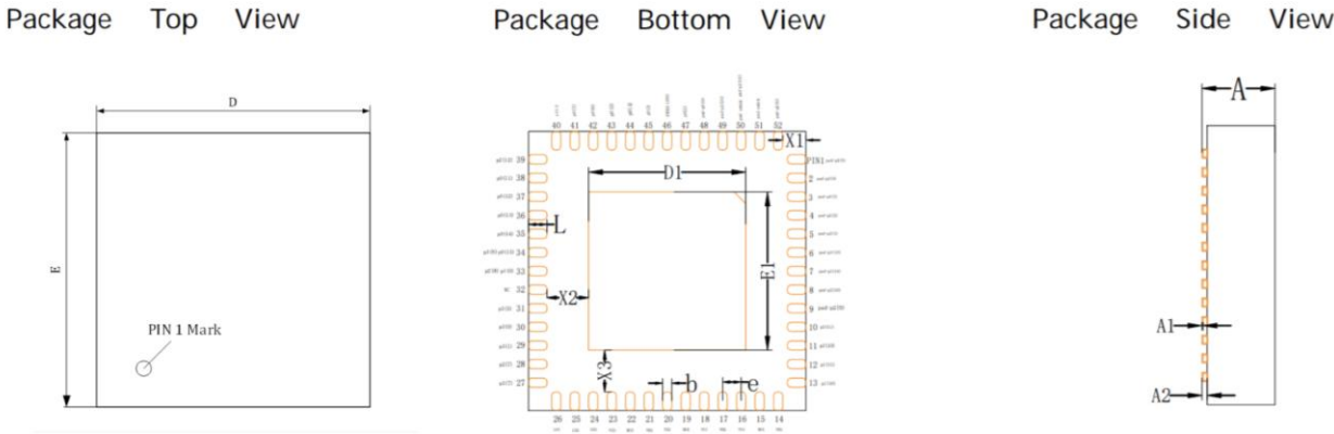
图 4-1 LKS32AT086N8Q9(B)封装图示
